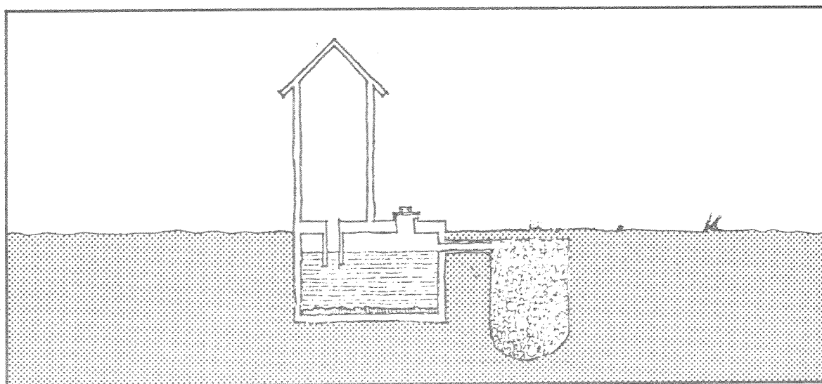
ACQUAPRIVY
