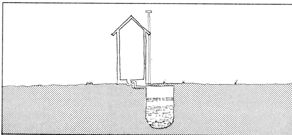
POUR-FLUSH TOILETS
